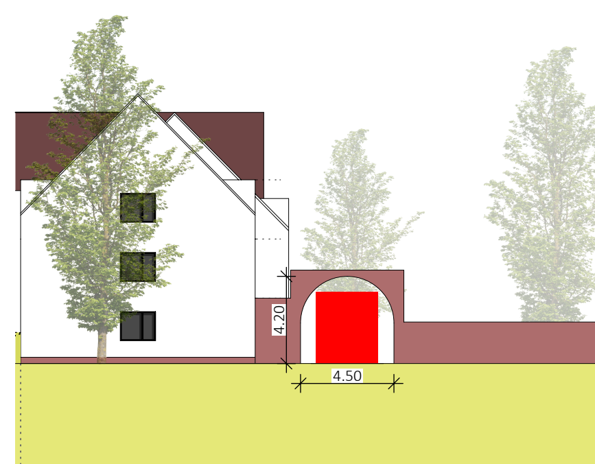
Durchfahrtsmaße Torbogen
